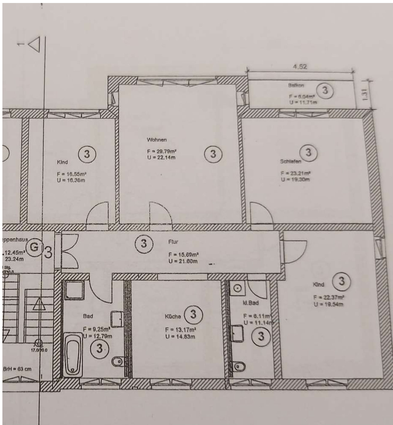
Grundrisskizze Whg. 3
